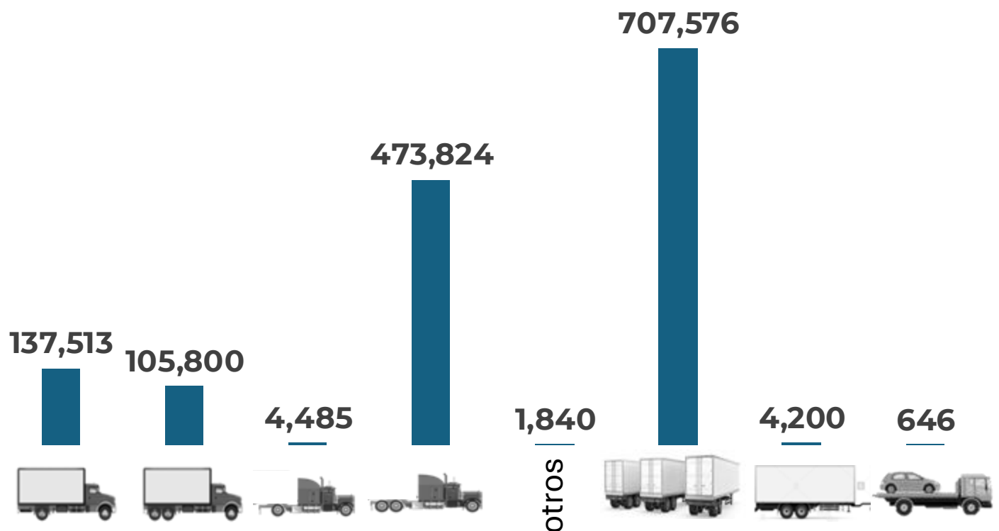
Composición del parque vehicular del autotransporte de carga
